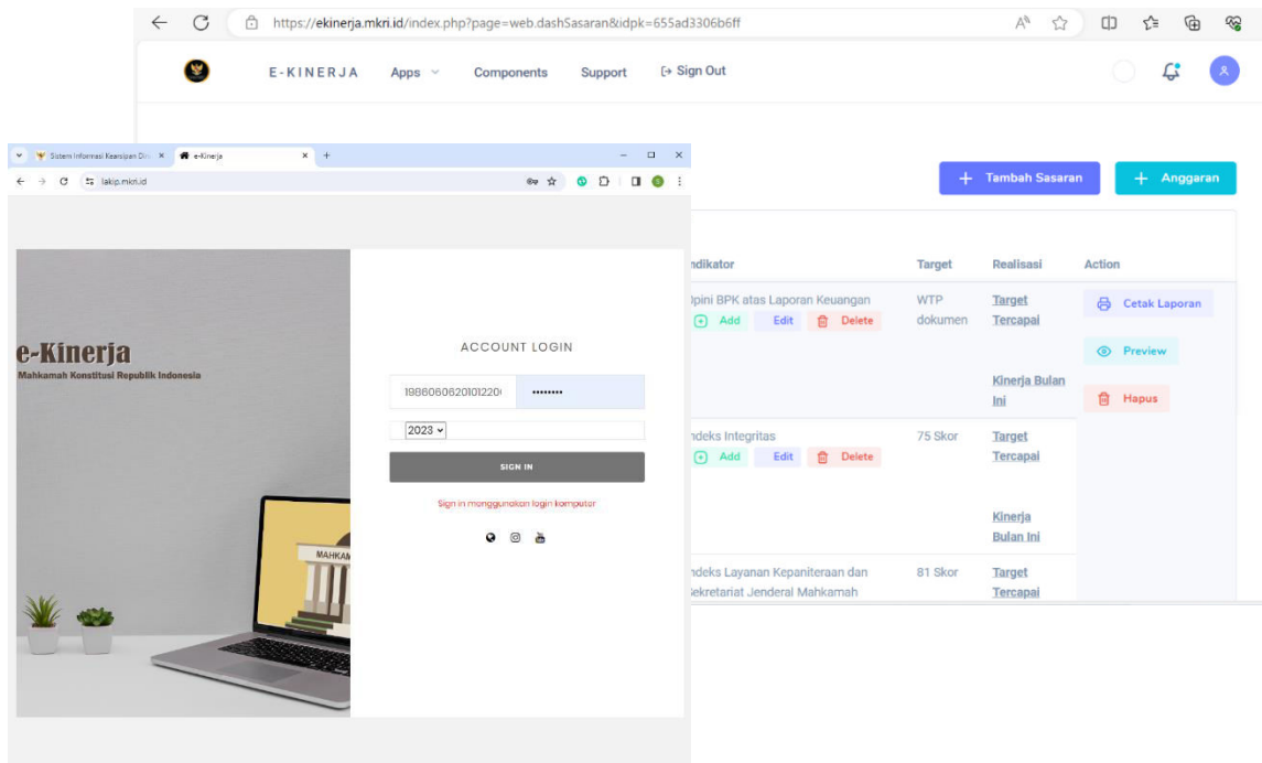
Gambar 7 Aplikasi e-Kinerja
